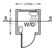
Toilet - Plan Scale - 1 : 100
